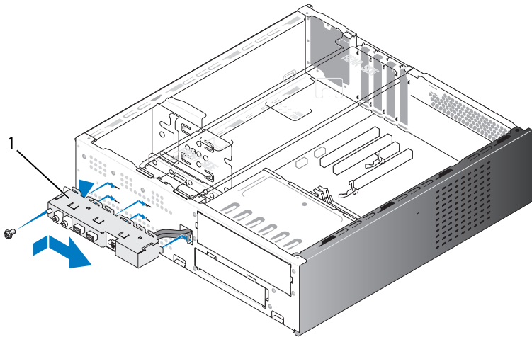
1 Panel de E/S
