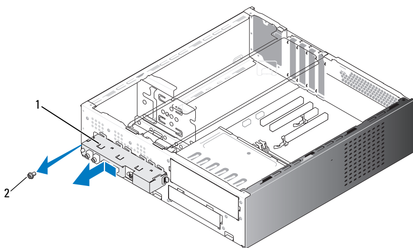
1 Panel de E/S 2 Tornillo
