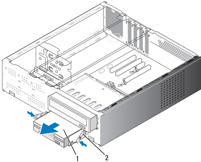
1 Unidad de disquete 2 Lengüetas elásticas (2)
