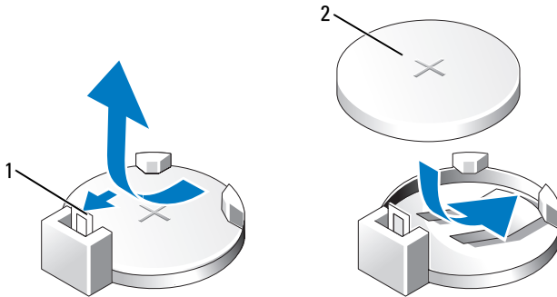
1 Palanca de liberación de la batería 2 Batería (polo positivo)
