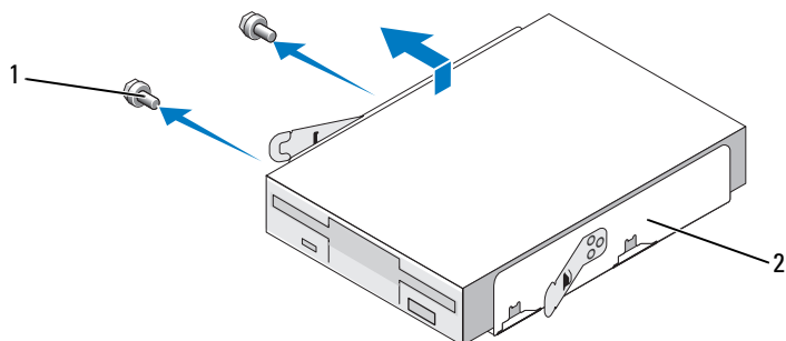
1 Tornillos (2) 2 Canastilla para unidades FlexBay
